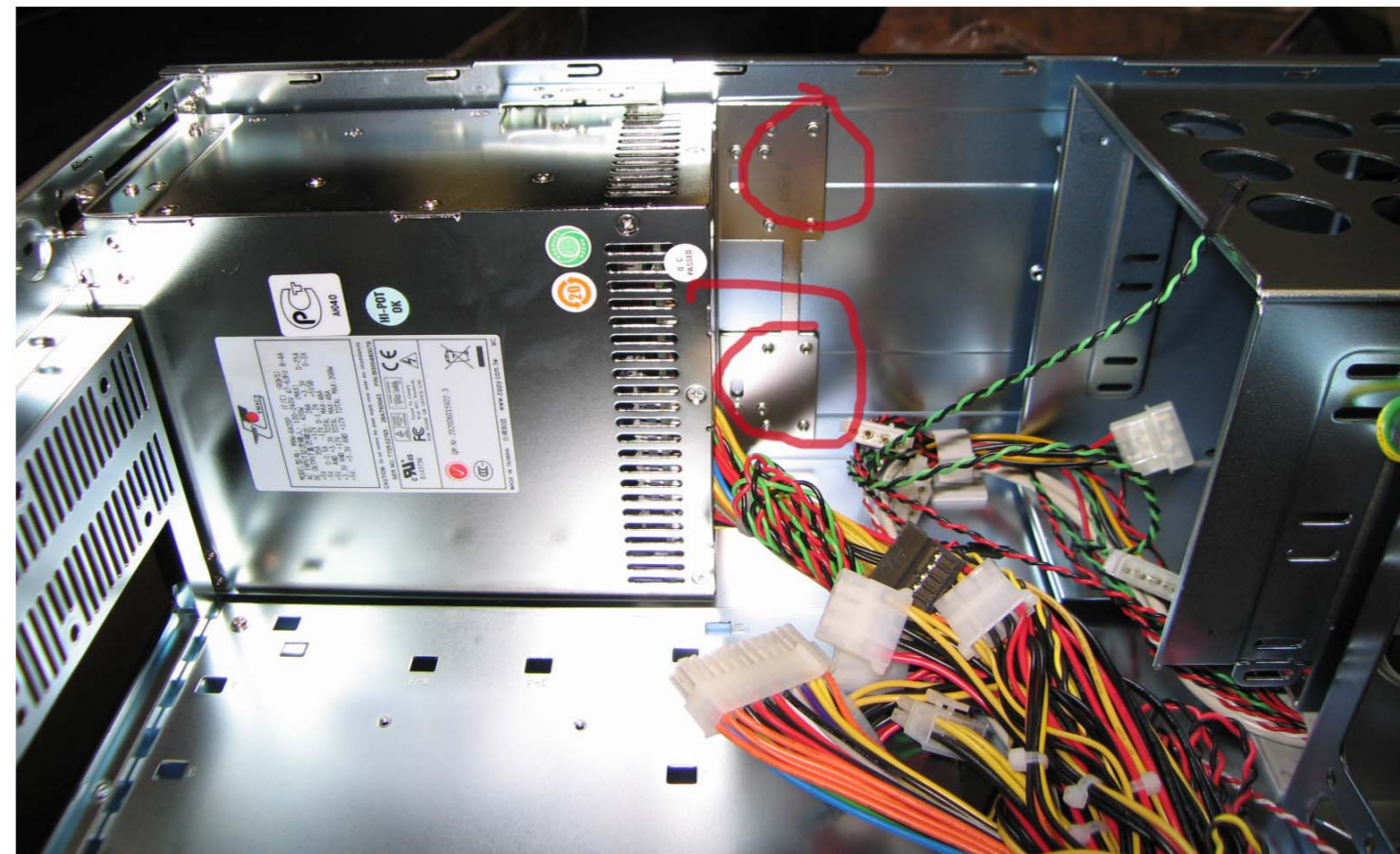
7. Das Netzteil einsetzen und verschrauben
